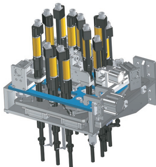
トランスミッションカバー締付機 (ピッチ可変機能付)
